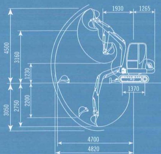
DIMENSIONS / ABMESSUNGEN / ГАБАРИТНЫЕ РАЗМЕРЫ M-28
