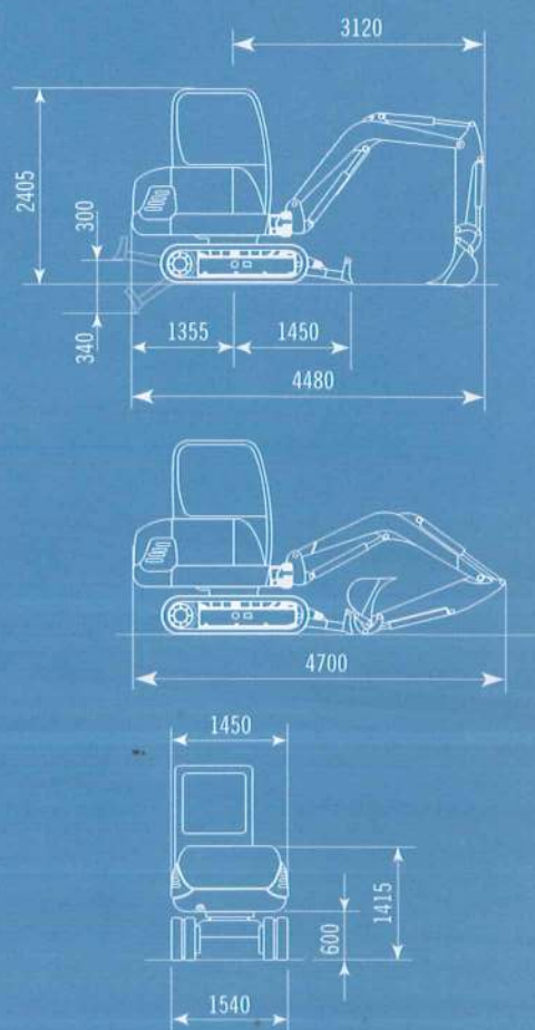
DIMENSIONS / ABMESSUNGEN / ГАБАРИТНЫЕ РАЗМЕРЫ M-35
