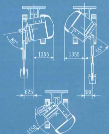
PERFORMANCES / LEISTUNGEN / ЭКСПЛУАТАЦИОННЫЕ ХАРАКТЕРИСТИКИ M-35
