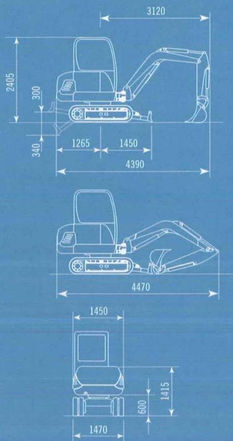
DIMENSIONS / ABMESSUNGEN / ГАБАРИТНЫЕ РАЗМЕРЫ M-28
