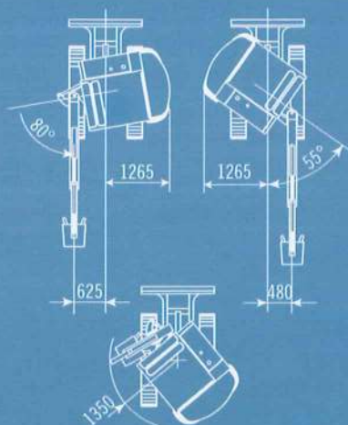
PERFORMANCES / LEISTUNGEN / ЭКСПЛУАТАЦИОННЫЕ ХАРАКТЕРИСТИКИ M-28
