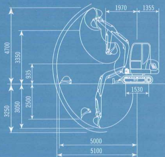
DIMENSIONS / ABMESSUNGEN / ГАБАРИТНЫЕ РАЗМЕРЫ M-35
