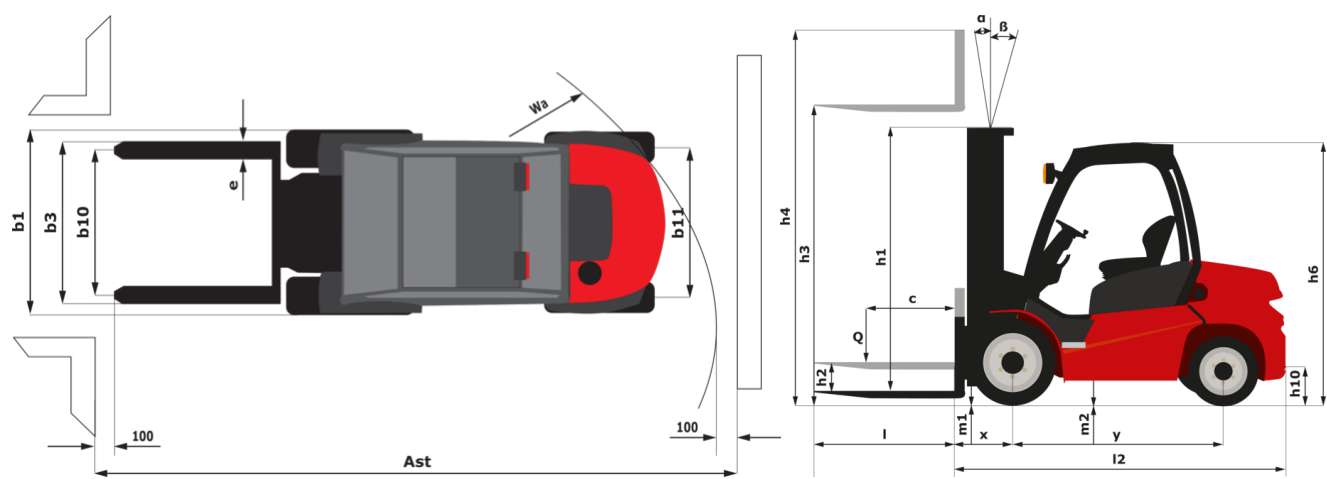
MSI 30 ST5 - Tekening met afmetingen
