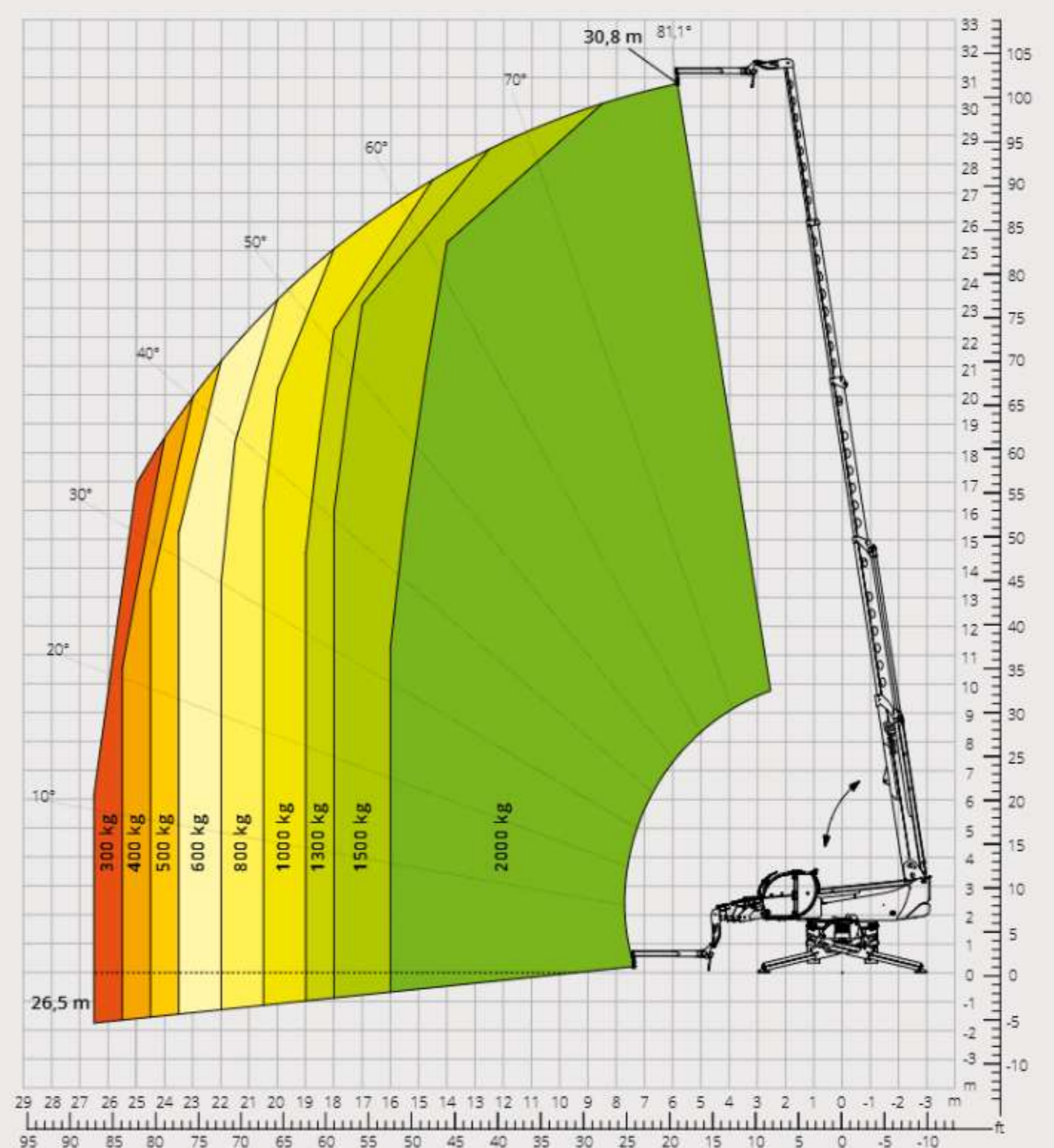
Load chart with JIB, 2,000 kg ATT - 04 - 013
