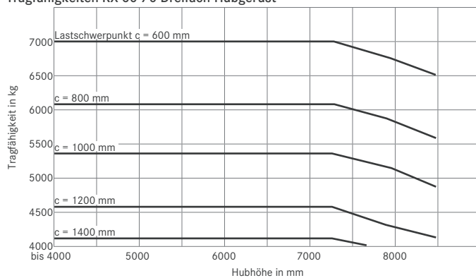
Tragfähigkeiten RX 60-70 Dreifach-Hubgerüst
