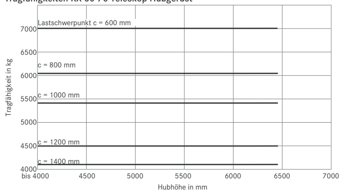
Tragfähigkeiten RX 60-70 Teleskop-Hubgerüst
