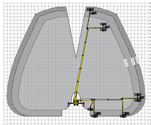
Arbeitskorblast 500 kg
