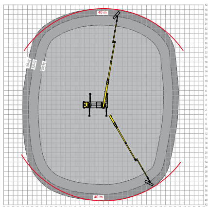
Arbeitskorblast 500 kg
