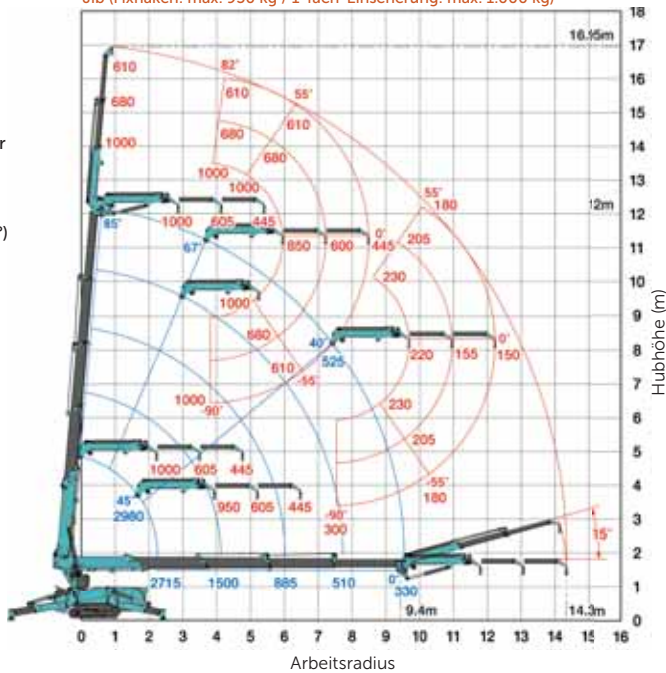
Dieses Arbeitsbereichsdiagramm zeigt die Gesamtlast einschließlich der Auslenkung des Auslegers.
