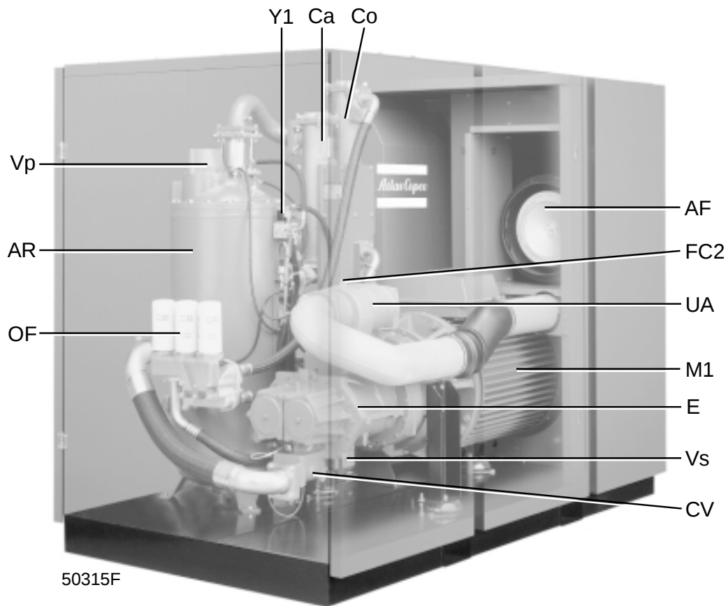
Fig. 1b GA110 W
